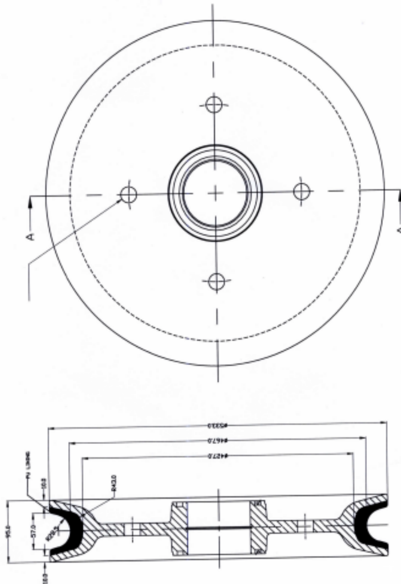
SECTION A-A
