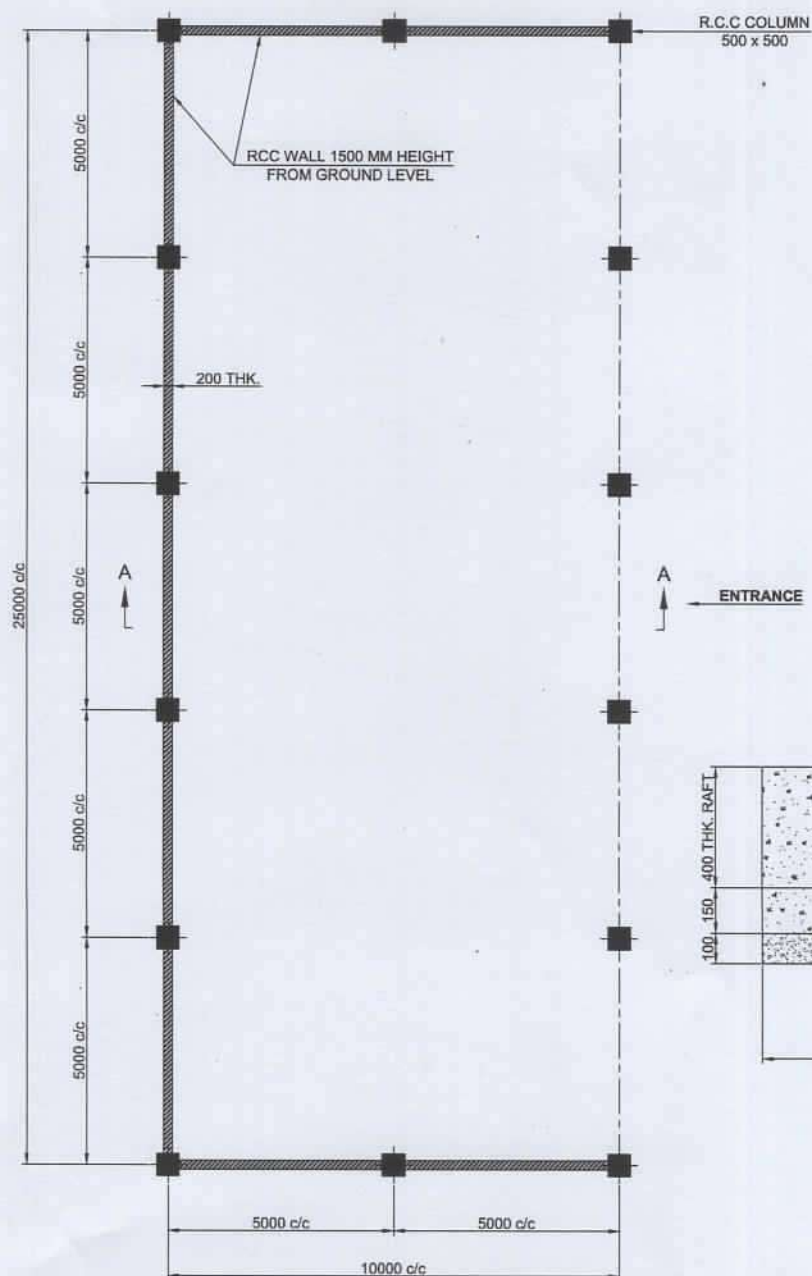
PLAN (SCALE - 1 : 80)
