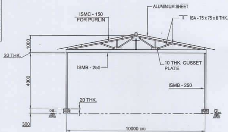
SECTION - AA (SCALE - 1 : 80)
