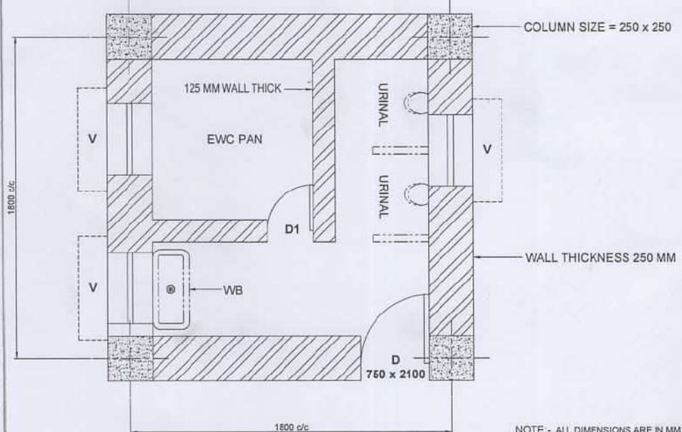
PLAN (SCALE - 1 : 12)
